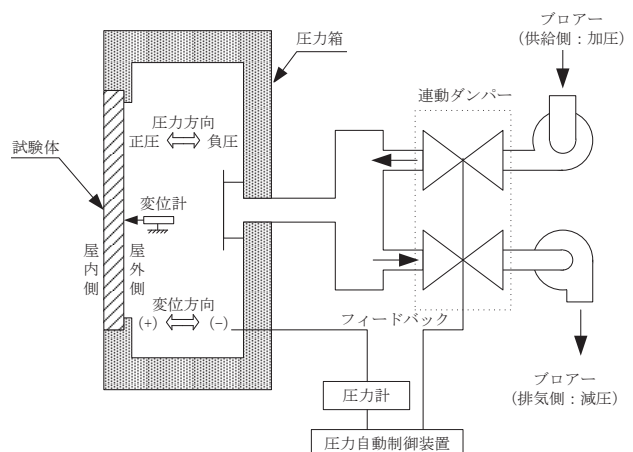
図1 動風圧試験装置の概要
