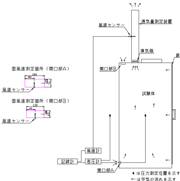
図1 試験概要図
