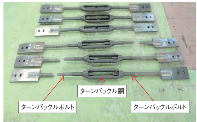
写真5 建築用ターンバックル
