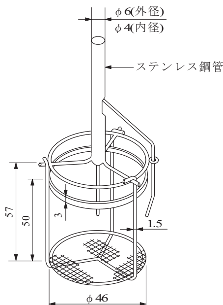
図2 試験体ホルダー(寸法単位:mm)
