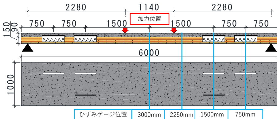
図1 試験体
