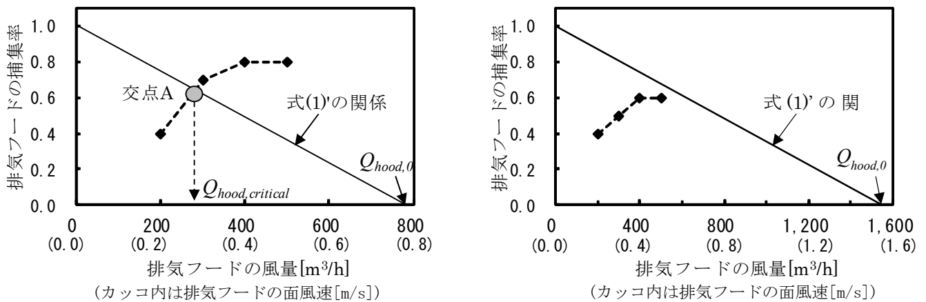
(1) 交点 A が排気フードの面風速 0.5m/s 以下で存在する場合
